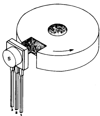
Dwg. A-12,574
