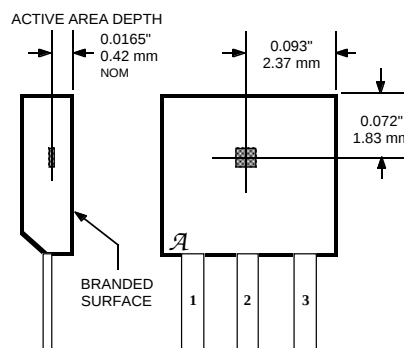
Dwg. MH-002-5D
